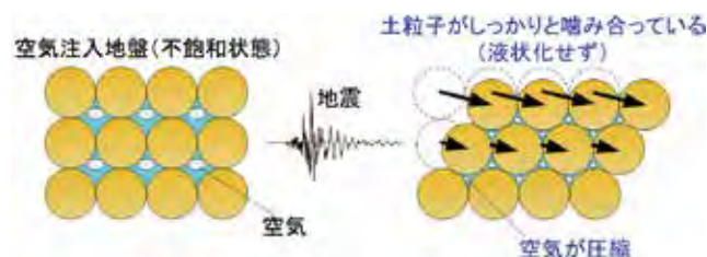
図-4 不飽和化した地盤の液状化強度増加メカニズム
