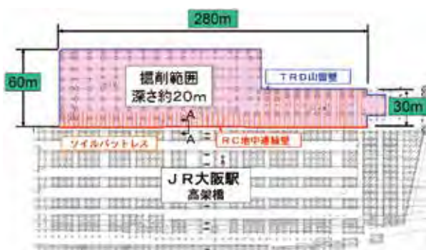
図-2 平面図
