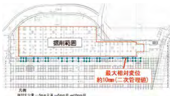
図-9 高架橋相対変位計測結果(平成22年12月24日)
