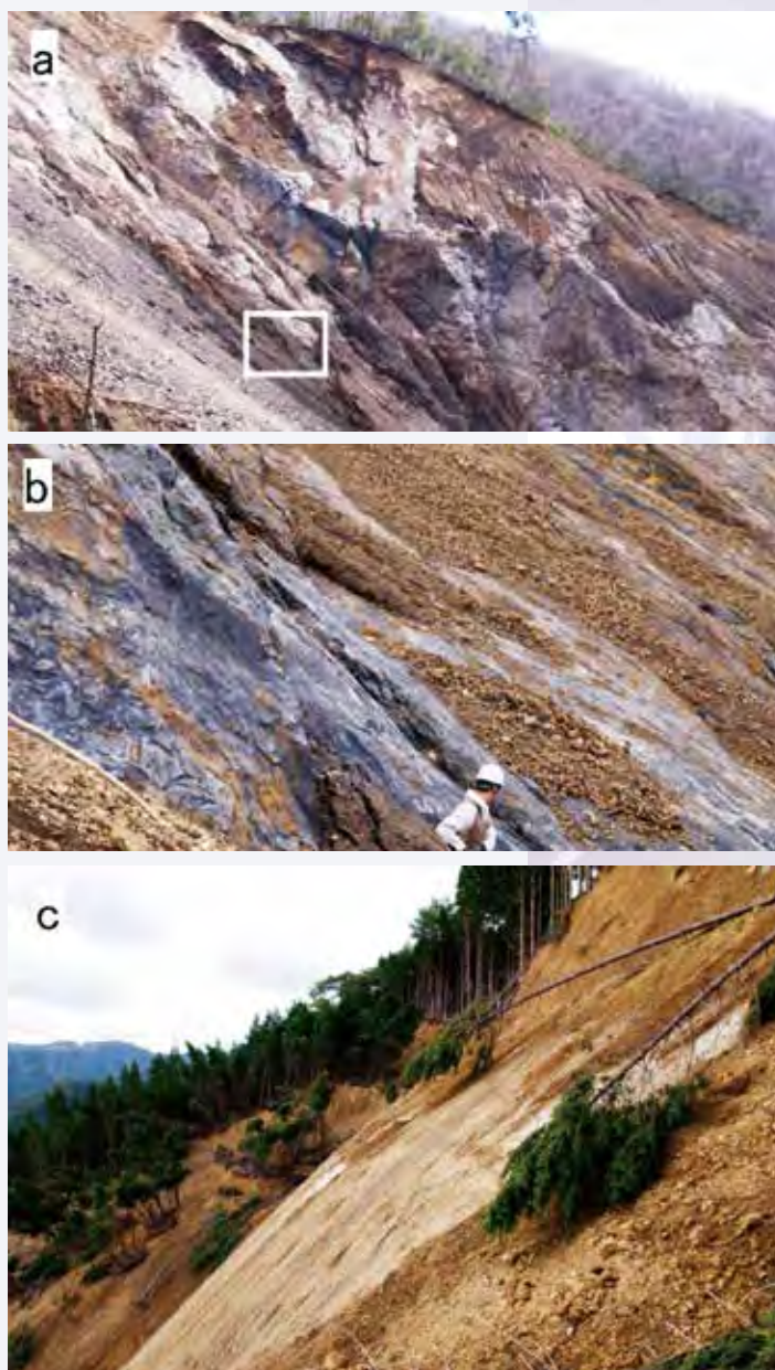
図-4 崩壊地に露出したせん断面。鏡肌を有し、湾曲・分岐・併合を繰り返す。 a: 赤谷の崩壊の向かって右上部。 b: aの四角内。岩石は混在岩。 c: 北股の崩壊最上部。
