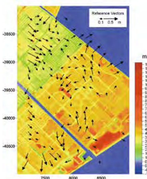
図-4 2011年東北地方太平洋沖地震で液状化が生じた東京湾岸の埋立地に見られる地盤の側方移動。2006年および2011年の地震前後の航空レーザ計測による1mDEMから計測。
