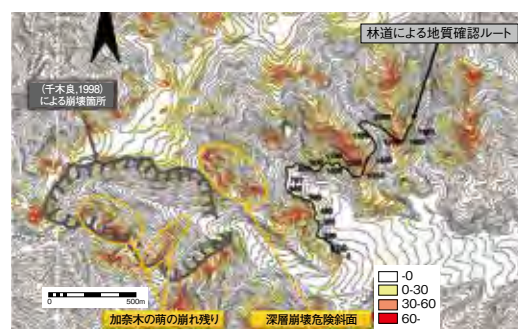
図-6 地震による崩れやすさおよび地形による地震動増幅効果を考慮した南海トラフ地震(300gal)による深層崩壊危険度
