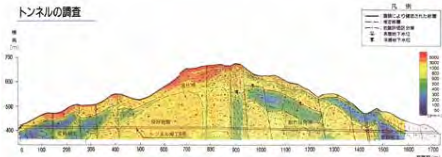
図-2 2次元電気探査の解析結果例（応用地質株式会社パンフレットより）
