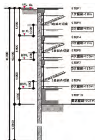
図-4 掘削の施工手順 (A-A断面)
