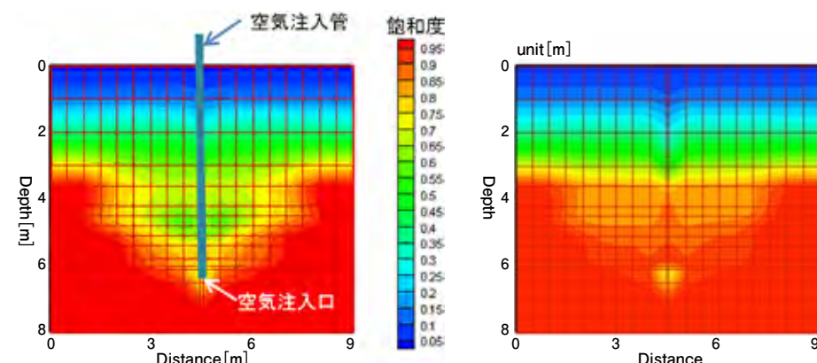
図-2 Air-des工法の空気注入中のイメージ
