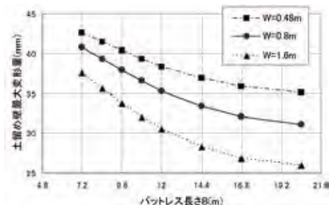
図-7 土留め壁最大変形量とバットレス長さの
