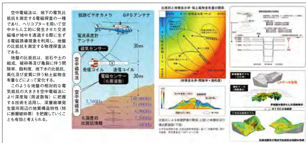
図-6 空中電磁法による深層崩壊発生に関連する地質構造の把握
