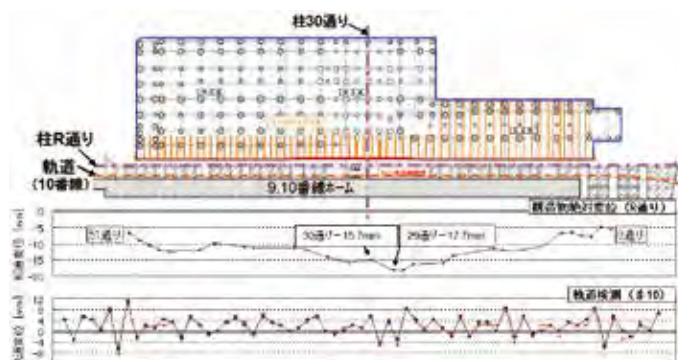
図-8 高架橋・軌道計測結果(3次掘削完了時)
