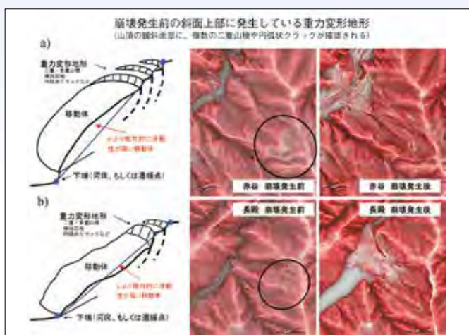
図-5 深層崩壊発生箇所での災害前に確認された斜面上部の重力変形地形
