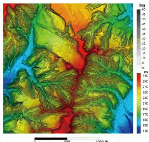
図-2 新潟県魚沼市の地すべり地帯を表現したELSAMAP。2004年の航空レーザ計測による2mDEMから作成。
