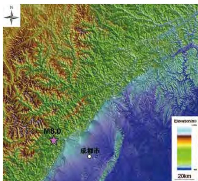
図-3 四川省成都市周辺の陰影起伏図。 スペースシャトルの3秒地形データSRTM-3を用いて作成（SRTM-3は、レーザ計測ではなくレーダ計測によるもの）。
