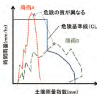
図-7 土砂災害の予測
