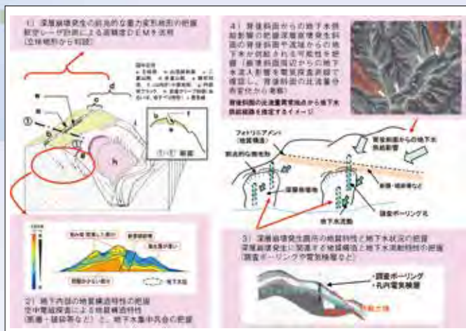
図-3 深層崩壊発生リスクの把握に向けた調査・検討の取り組み
