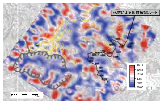
図-5 岩盤の緩みの著しい斜面を表示した比抵抗凹凸度分布
