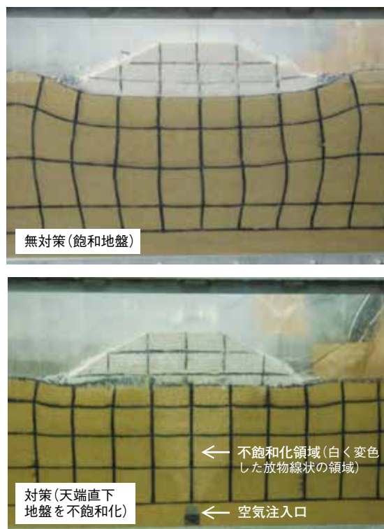
図-6 遠心模型実験による不飽和化の効果の検証。加振後の変形状況。
