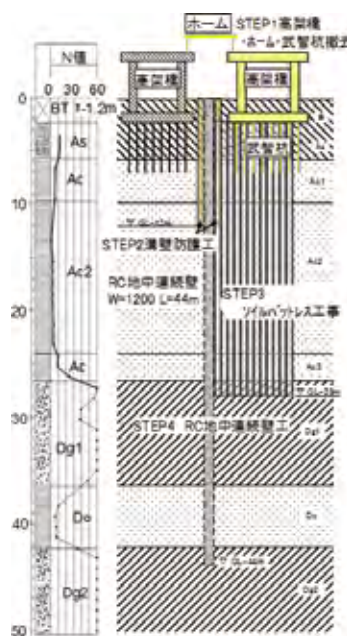
図-3 土留め壁施工手順
